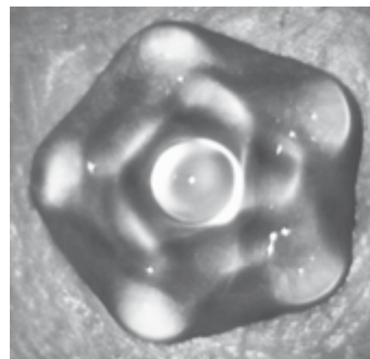
Schwingender Wassertropfen
